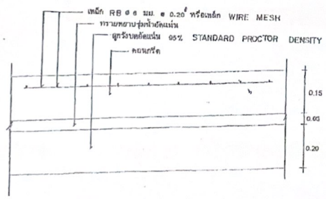
รายละเอียดบริเวณรอยกั๊ตเสริมเหล็ก
