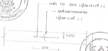
LONGITUDINAL JOINT
