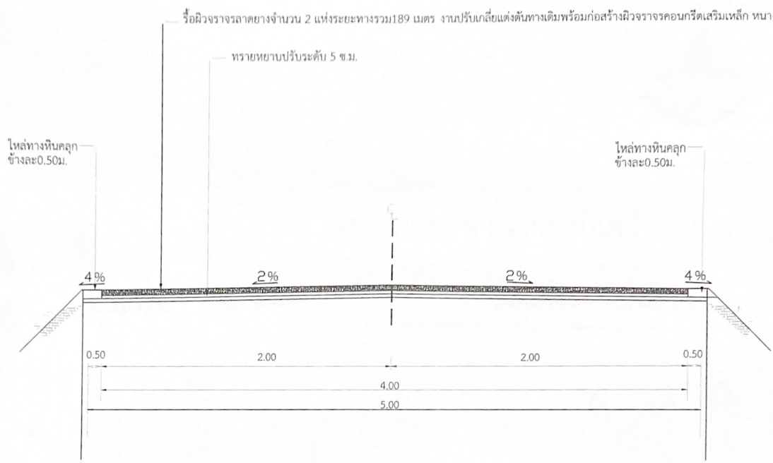
รูปตัดถนนคอนกรีตเสริมเหล็ก หนา 15 ซม. มตข.ระบ. NO SCALE
