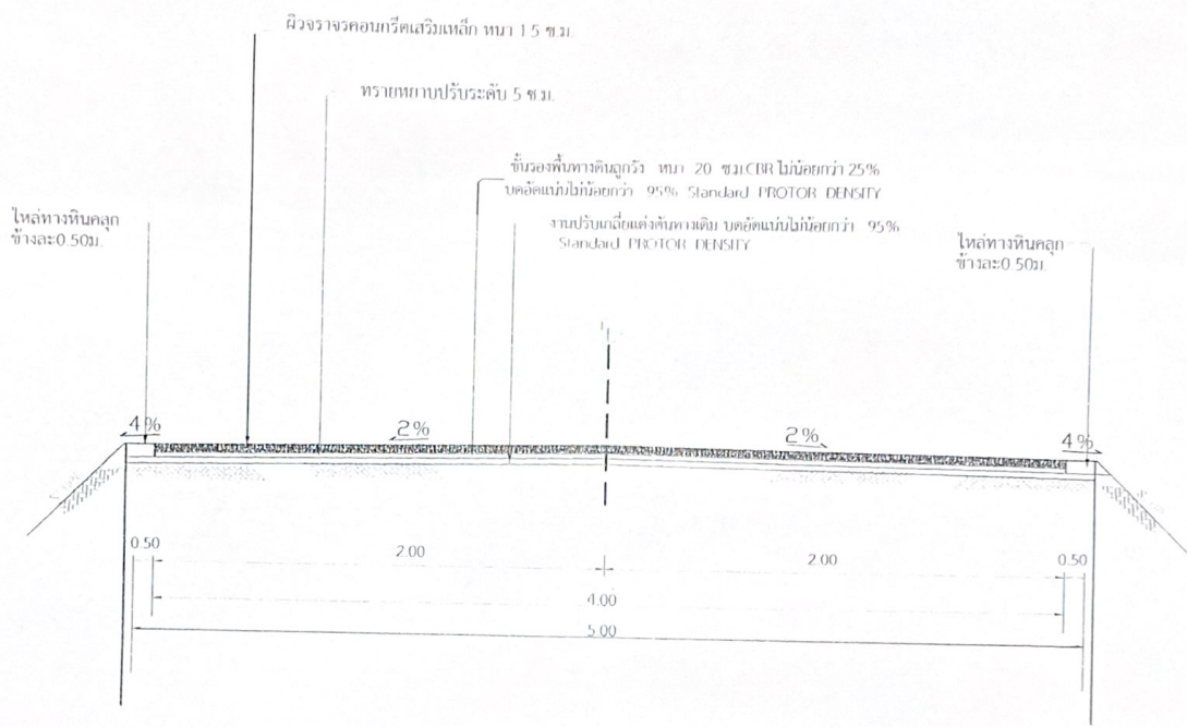
รูปตัดถนนคอนกรีตเสริมเหล็ก ทหนา 15 ซม. ม.ช.ร.ม. NO SCALE
