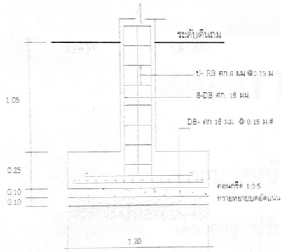
ขยาย F1,C1
