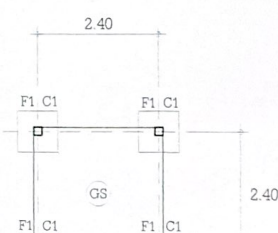
แปลนโครงเหล็กคานตั้ง
