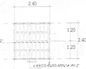
แปลนโครงเหล็กคานตั้ง
