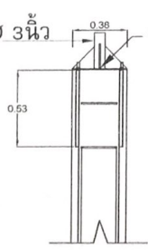
ขยายแผ่นเหล็กรองหัวเส้า
